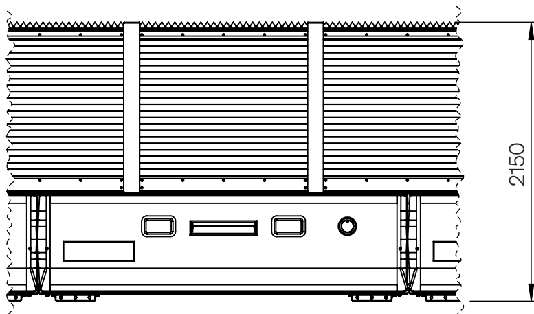
Basisutførelse
